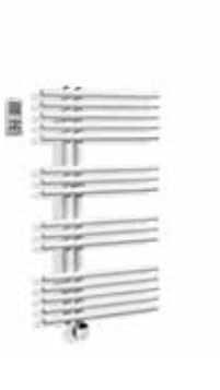
596 500 – 596 501 Badheizkörper Pavone E, Öffnung rechts, Anschluss elektrisch 230 V, Heizstab links, Infrarot Thermostatsteuerung SP1, IP44, Fernbedienung programmierbar, Befestigungsmaterial 596 500: 51 x 85,6 cm, 700 W 596 501: 61 x 85,6 cm, 700 W
